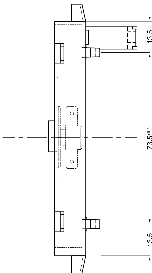
BASE de BORNERA ARMADA
